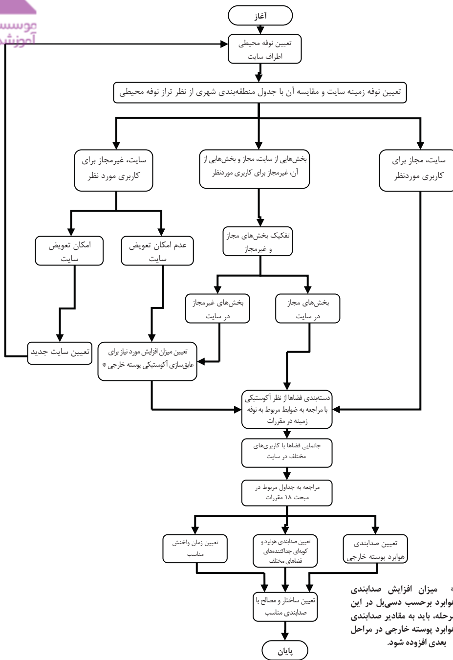
شکل پ-۱: دیاگرام مراحل مختلف طراحی آکوستیکی یک ساختمان
