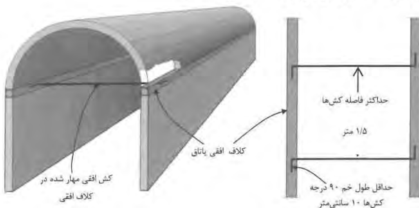
شکل ۷-۳۱ تعبیه مهاربند افقی در پاتاق قوسی استوانه‌ای
