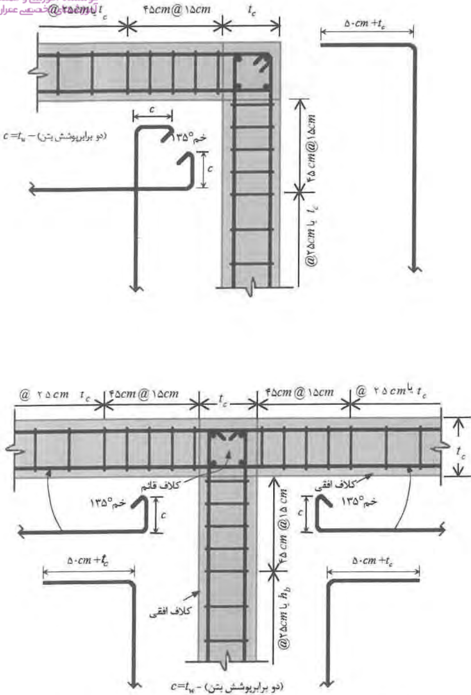
شکل ۱۷-۷. جزئیات اتصال دو کلاف برای بارهای منفی و مثبت
