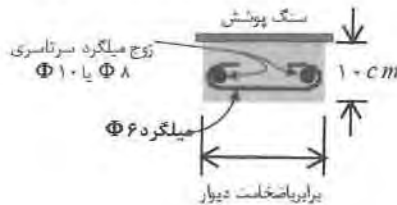
شکل ۷-۱۶ جزئیات مهار جان‌پناه
