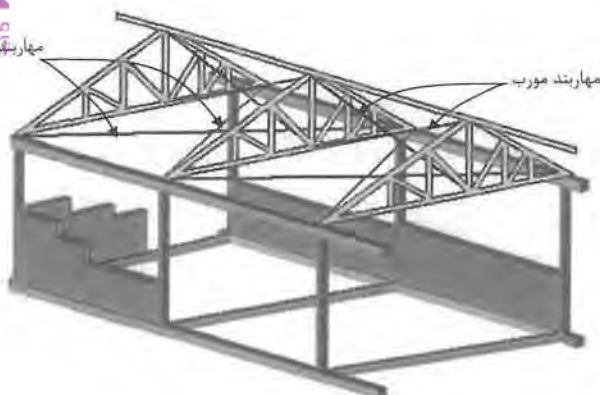
شکل ۷-۳۰ تعبیه مهاربندهای قائم و افقی در خرپاها
