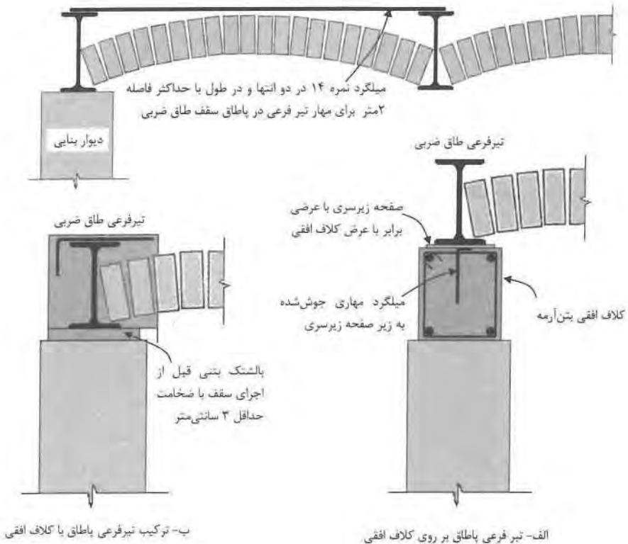
شکل ۷-۲۸ جزئیات منسجم کردن تیرآهن‌های سقف طاق ضربی
