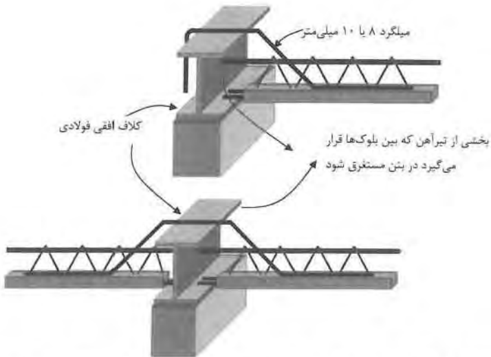
شکل ۲۹-۷ نحوه اتصال تیرچه‌های سقف به کلاف افقی بتنی و فولادی
