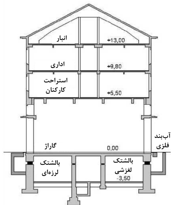
مقطع عرضی ساختمان به همراه بالیستک‌های لرزه‌ای در زیرزمین (بچمن و زچمن، ۲۰۰۸)
