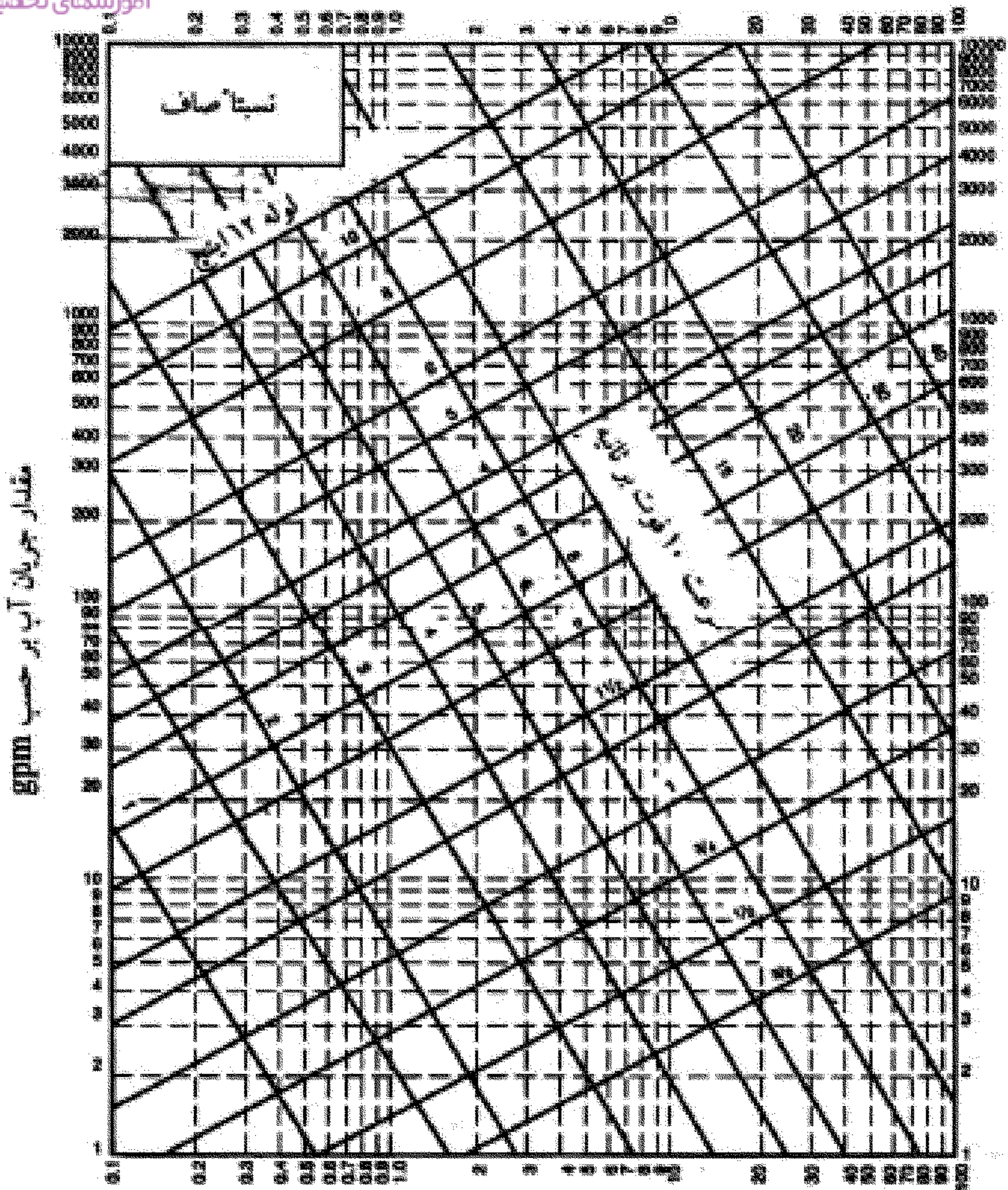
ارتفاع فشار آب بر حسب پوند بر اینچ مربع در ۱۰۰ فوت طول
