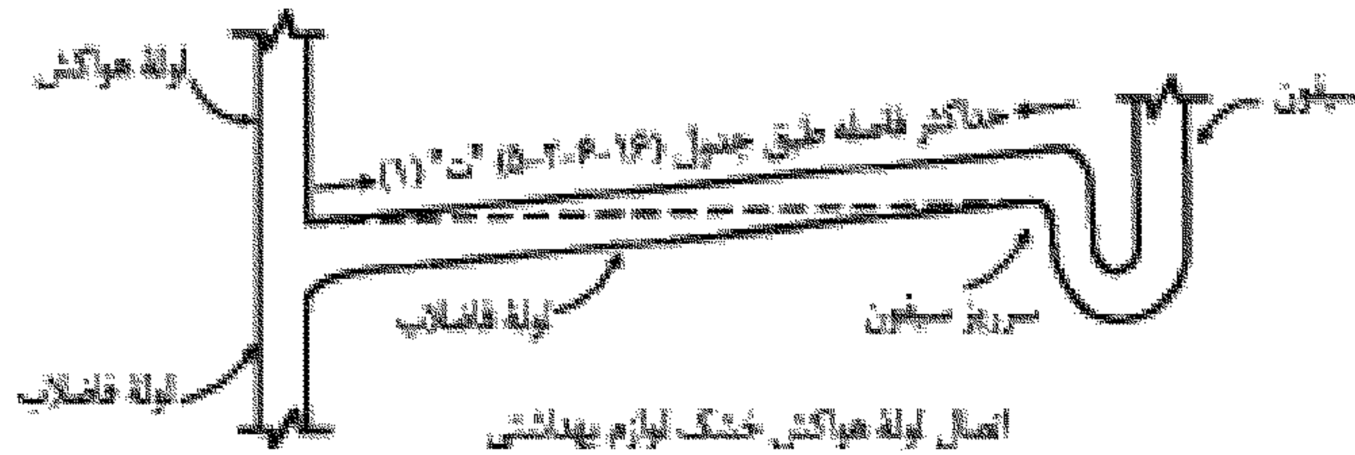
شکل شماره (۱۶-۶-۲-۵) ت" (۱): اتصال لوله هواکش خشک لوازیم بهداشتی
